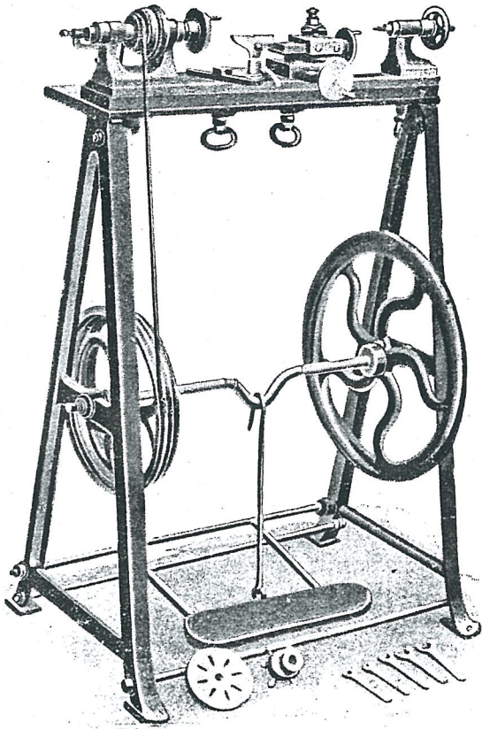
Šlapací soustruh
